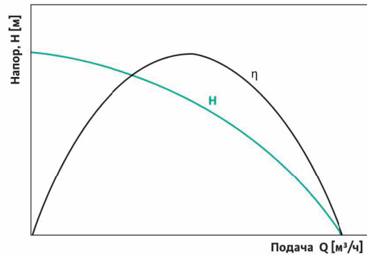
Характеристика насоса и кривая КПД на графике Q–H
