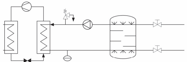
Конденсатор Испаритель
